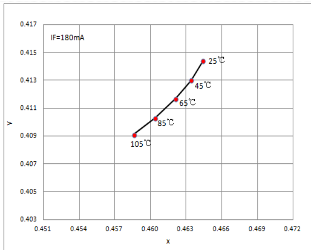
Fig 9. Ts vs. CIE x, y Shift
