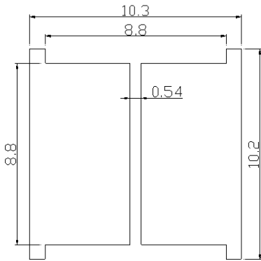
建议焊盘
